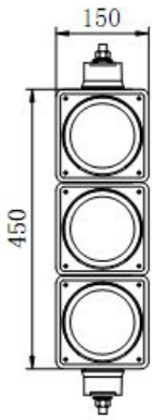
Elevation
